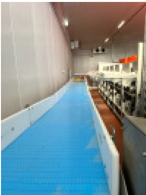
ALCO Chargieranlage Typ ASL 1000-3 Laufnummer: 12130 Preis: € 150.000,-
