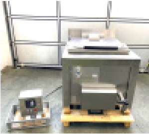
FESSMANN Kesselanlage NOVA 300I Gas Laufnummer: 10320 Preis: € 9.500,-
